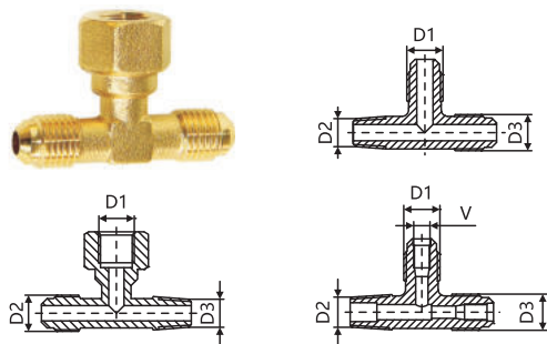
三通接头 (异径) Reducing Tee
