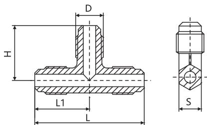
三通接头 (异径) Reducing Tee
